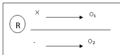
Gambar 1. Desain Penelitian
