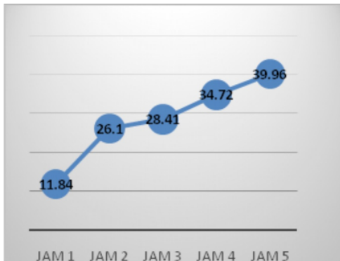
Gambar 1. Grafik nilai penurunan kekeruhan setelah perlakuan selama 5 jam
